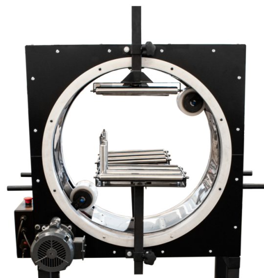
EP-6700-25 Envolvedora de Anillos Motorizada - 630 mm
